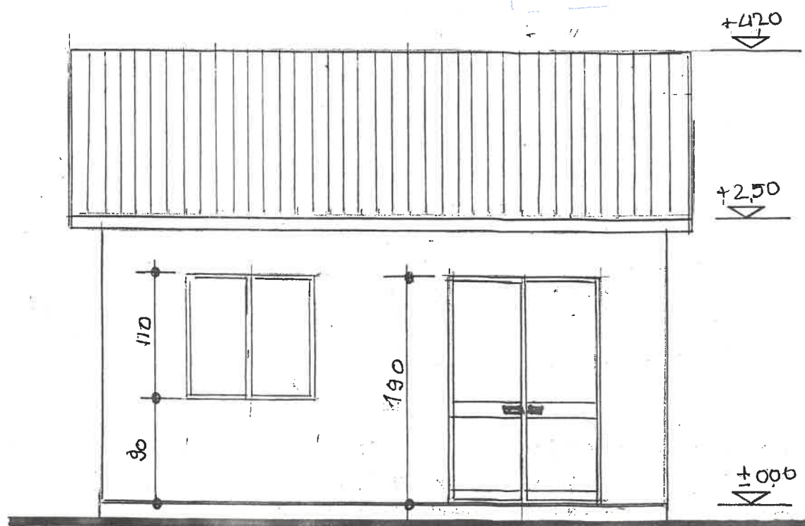
FATAȚA PRINCIPALĂ - CORP C1
