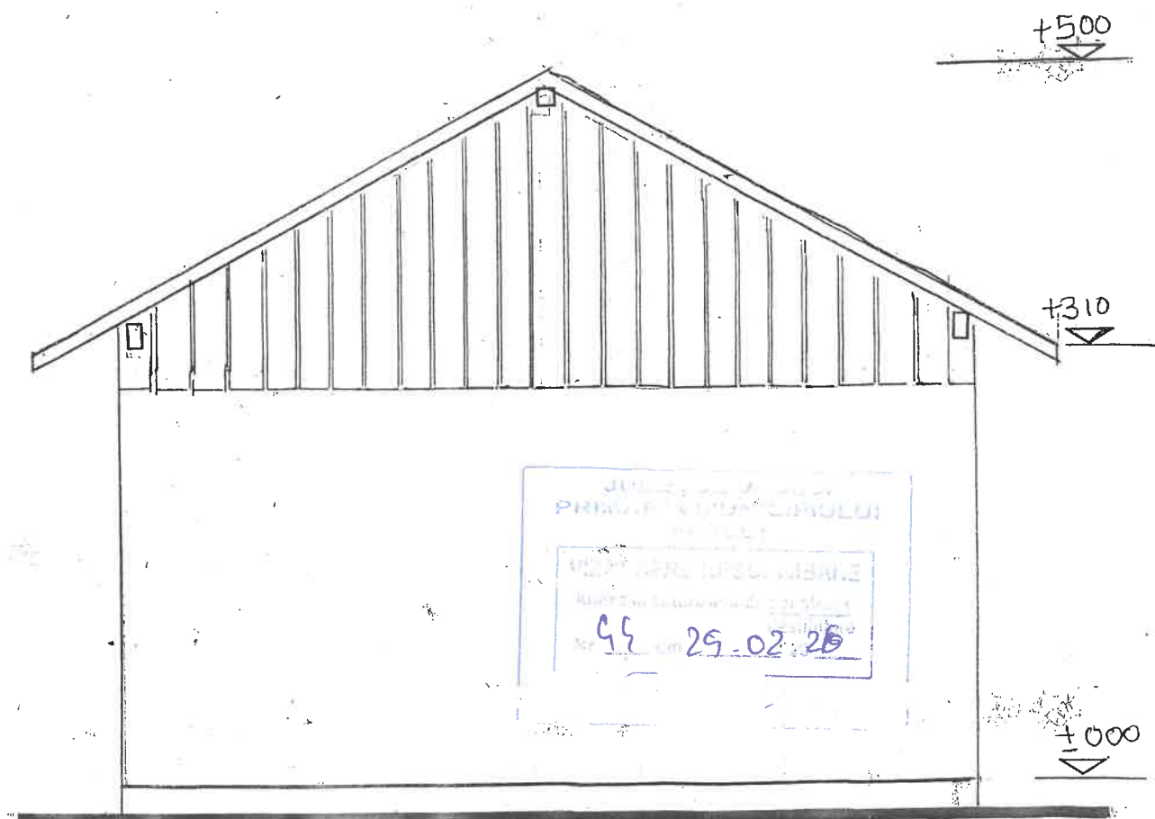
FATADĂ LATERALĂ STÂNGA CORP C3
