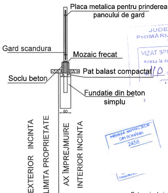
SECȚIUNEA A-A
