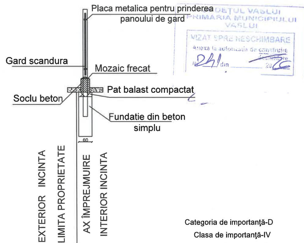
SECȚIUNEA A-A
