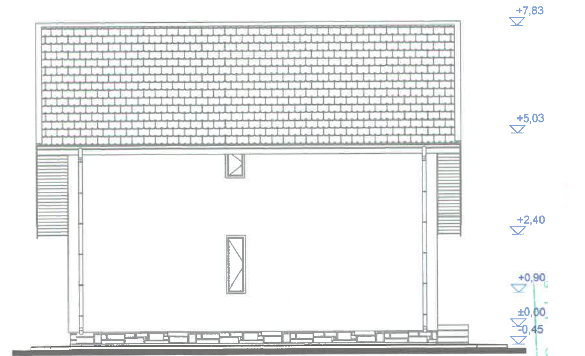
FATADA LATERALA DREAPTA 1:100
