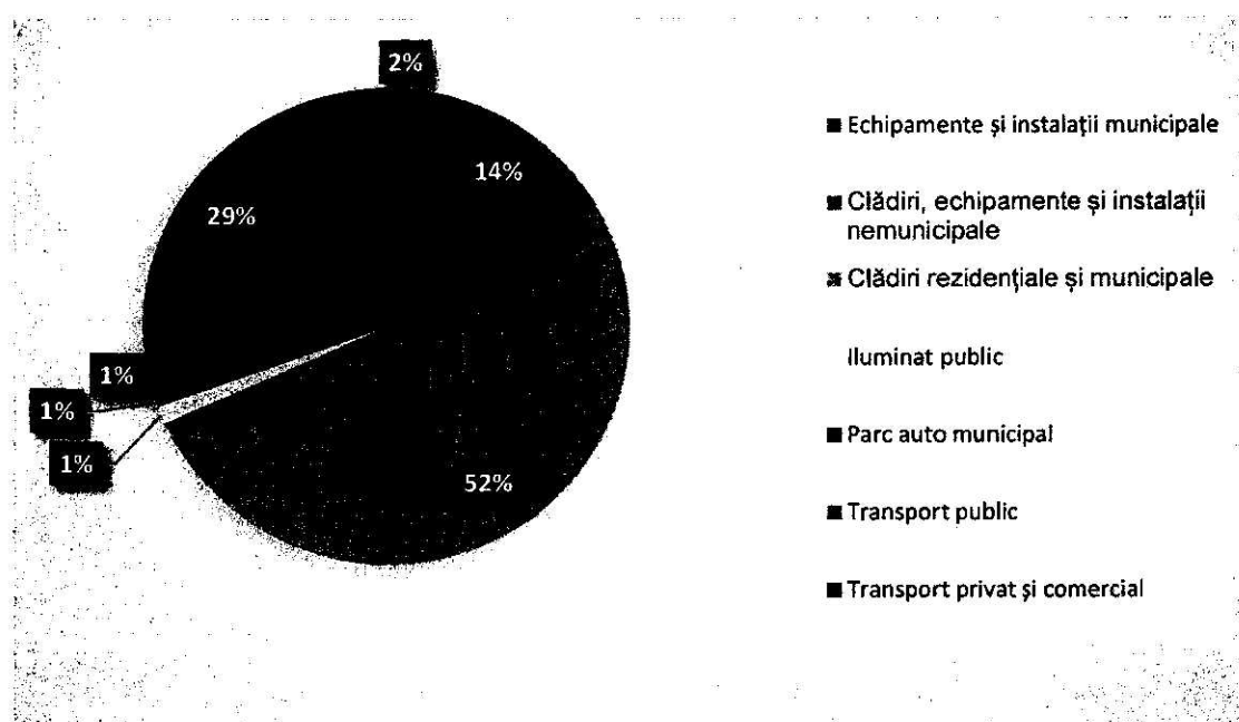
Figură 45 - Emisiile de CO 2 de la nivelul municipiului Vaslui, pe sectoare, în anul 2009
